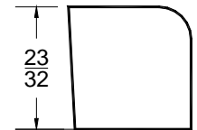
FLUSH DOORLITE MOULDING #300
