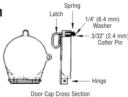
Door Cap Cross Section
