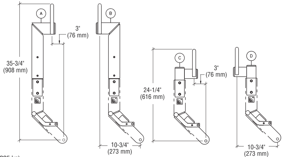
CAT. NO. LB6ALO
