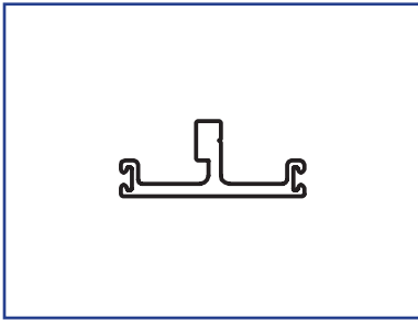
US01-0611-LLCL UniSlide Telescopic Lower Edge US01-0611-LLDB UniSlide Telescopic Lower Edge
