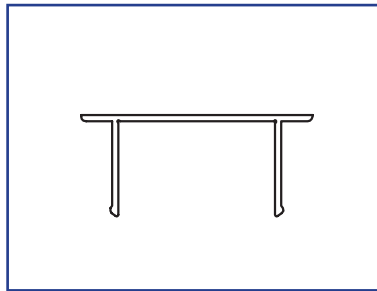
US01-0933-LLCL Redesigned Jamb Filler US01-0933-LLDB Redesigned Jamb Filler
