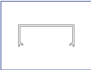
US01-0463-LLCL Bi-Way Jamb US01-0463-LLDB Bi-Way Jamb
