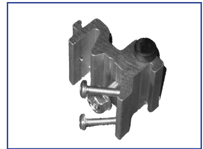
US05-0600-02 Door Stop Kit, RH US05-0600-01 Door Stop Kit, LH
