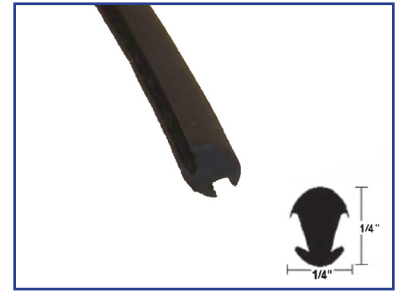
US20-0213-01 Vyram Rubber Glass Bead
