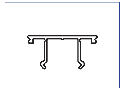
US01-0430-LLCL Jamb Closure US01-0430-LLDB Jamb Closure
